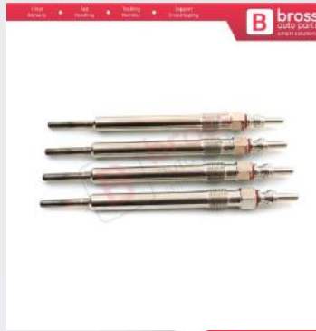
BGP95-1 Audi Seat Skoda VW için 4 Adet Kızdırma Bujisi 4.4 Volt 03L963319 059963319F
