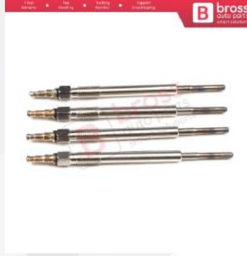
BGP14-1 VW Skoda Seat Audi Jeep için 4 Adet Isıtma Bujisi N10579802
