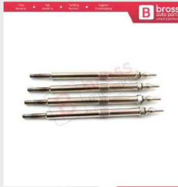
BGP90-1 Nissan Opel Renault İçin 4 Adet Kızdırma Bujisi 11 V 8200012099 4430069
