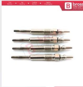
BGP103-1 Audi Seat Skoda VW İçin 4 Adet Kızdırma Bujisi 7 Volt N10591608
