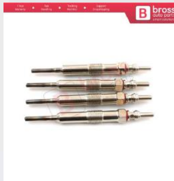
BGP104-1 Renault Dacia Mercedes Nissan 1.5 dCi Motor için 4 Adet Kızdırma Bujisi 4.4 Volt 8200682592
