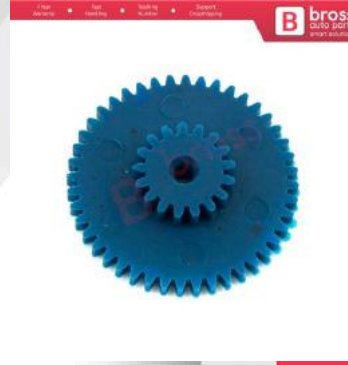
BGE653 Kilometre Sayaç Km/h VDO Hız Gösterge Tamir Dişlisi 44x17 Diş
