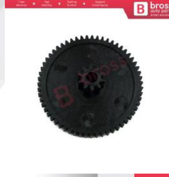
BGE685 BMW Mini One Cooper İçin EGR Valf Tamir Dişlisi 59/10 Diş
